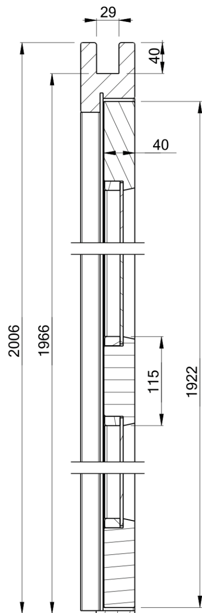
B-B
